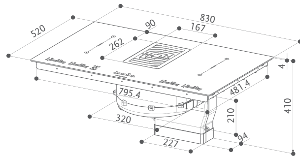
Montaža u režim filtracije sa prednjim odvodom za vazduh
